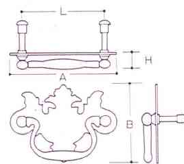
CC-13 [No.201] 材質/真鍮 仕上/本磨・古代色
