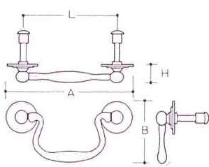
CC-12S [エイト鉄] 材質/ZAC 仕上/銅ブロンズ
