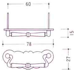
CC-14 [No.758] 材質/真鍮 仕上/古代色
